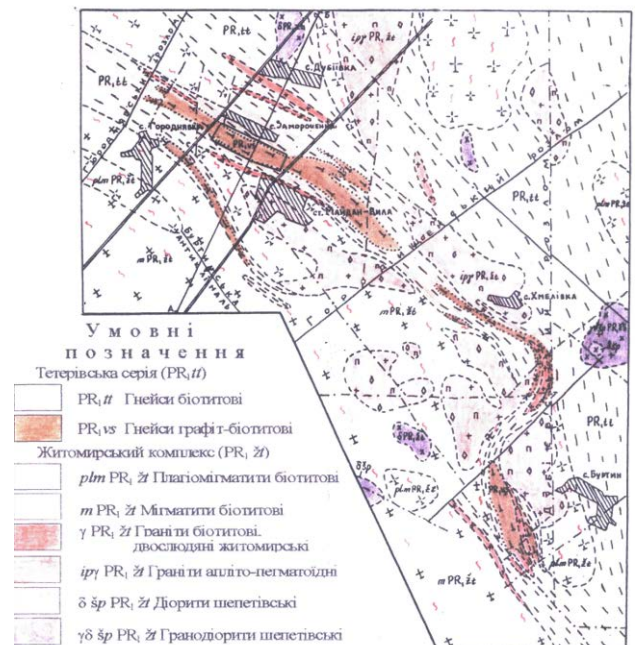
Геологічна карта кристалічного фундаменту Буртинського родовища графітових руд Масштаб 1: 100 000
